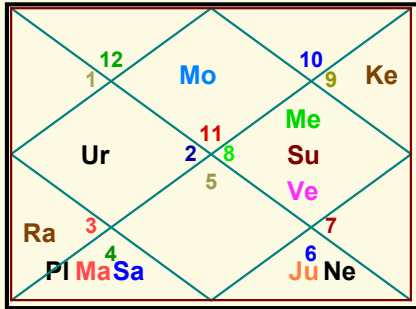
Lagna/Rashi Chart
