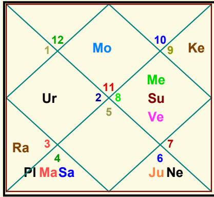
Lagna/Rashi Chart
