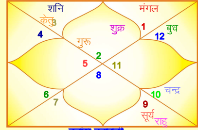
नवांश कुण्डली
